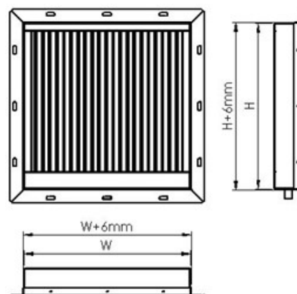
Skiss av CamVane AL WxHx100-DU FAR
